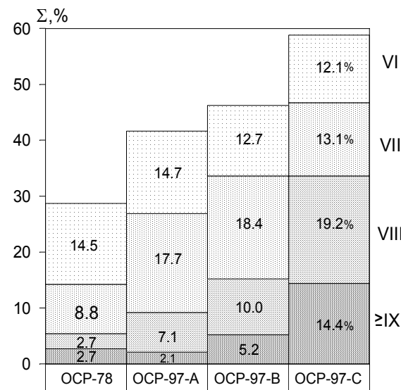
Рис. 11. Соотношения размеров площадей (% внутри прямоугольников) зон сейсмической интенсивности (римские цифры справа) на картах ОСР-97 (А, В, С) и ОСР-78. Шкала ординат отражает суммарные площади с сейсмической интенсивностью, превышающей VI, VII, VIII и \geq IX баллов.
