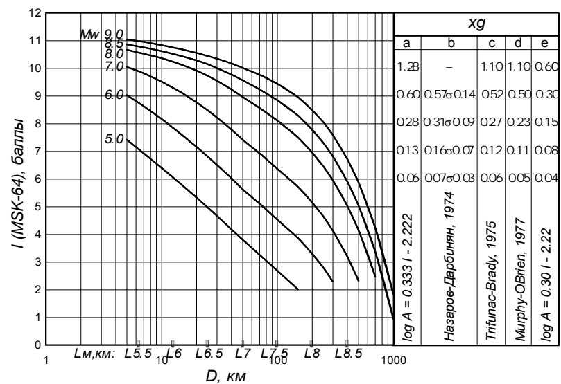
Рис. 9. Графики спадания балльности I с расстоянием D (км) от сейсмических очагов протяженностью L_m землетрясений разных магнитуд M_w (слева) и соотношения интенсивности I (MSK-64) с пиковыми ускорениями PGA колебаний грунта в долях ускорения силы тяжести g , по данным разных авторов: а – зависимость, принятая в ОИФЗ при создании карты Северной Евразии по программе GSHAP [57] в параметрах PGA ; с – зависимость, используемая в ряде европейских стран; авторы остальных соотношений указаны в таблице; в столбце b приведена величина стандартного отклонения \pm\sigma .
